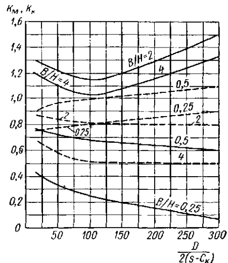
Рис. 29.8. Графики для определения коэффициента K при определении расчетных сил P'_m и P'_K , действующих на стенку цилиндрического корпуса при прямоугольной форме лап: — — — — K_m ; — — — — K_K
