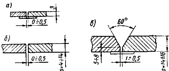
Рис. 10.12. Конструктивные элементы подготовки кромок листового титана и титановых сплавов толщиной 3—16 мм под стыковую автоматическую сварку под слоем флюса (по ОН 26-01-71—68): а — без разделки кромок, с подкладкой; б — без разделки кромок, без подкладки; в — V-образная разделка кромок, с подкладкой
