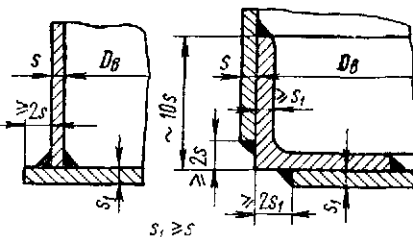
Рис. 16.13. Основные типовые конструкции плоских круглых днищ для аппаратов, работающих под наливом и атмосферным давлением
