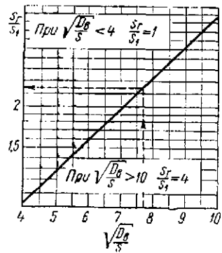
Рис. 21.14. График для определения толщины конической горловины во фланцах
