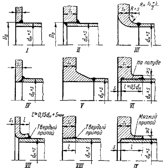
Рис. 19.5. Основные типовые конструкции неразъемного присоединения труб к различным частям аппаратов:
