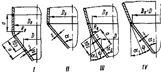
Рис. 16.10. Типовые конструкции конических днищ в сварной аппаратуре: I и III — с отбортовкой; II и IV — без отбортовки
