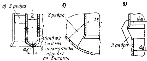
Рис. 31.13. Основные конструктивные узлы сварных барботеров типа газлифта: а — концевая часть газовой трубы; б — нижнее крепление подъемной трубы газлифта; в — крепление подъемных труб газлифта между собой
