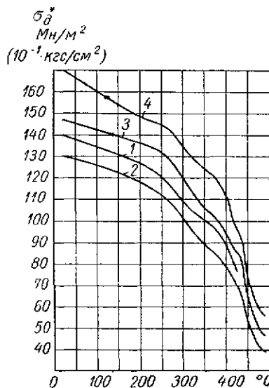
Рис. 14.1. Номинальные допускаемые напряжения \sigma_d^* для наиболее распространенных в химическом аппаратостроении марок углеродистой и низколегированной стали. Марка стали: 1 — Ст. 3; 2 — 10; 3 — 20 и 20К; 4 — 09Г2С и 16ГС
