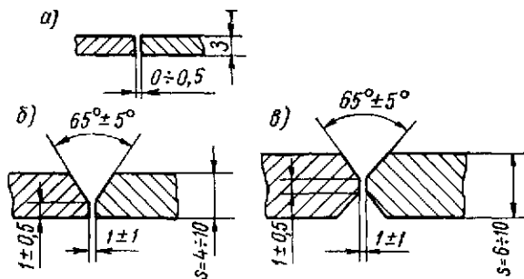
Рис. 10.9. Конструктивные элементы подготовки кромок листового никеля марки НП2 под стыковую ручную аргано-дуговую сварку (по ОН 26-01-71—68): а — без разделки кромок; б — V-образная разделка кромок; в — X-образная разделка кромок
