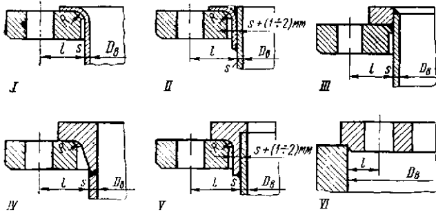
Рис. 21.17. Основные типовые конструкции свободных фланцев, применяемых в химическом аппаратостроении: I — при p_c \leq 0,6 Мн/м 2 на отбортовке из пластичных материалов; II — при p_c \leq 0,6 Мн/м 2 и s \leq 15 мм из меди и латуни на приварном бурте из стали; III — при p_c \leq 0,6 Мн/м 2 на приварном бурте из стали; IV — при p_c \geq 2,5 до 20 Мн/м 2 на приварном бурте из стали и при p_c \leq 1 Мн/м 2 — на приварном бурте из алюминиевых сплавов; V — при p_c > 0,6 до 5 Мн/м 2 на приварном бурте из латуни; VI — на цилиндрической опорной поверхности
