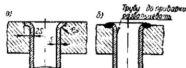
Рис. 10.14. Приварка труб к трубным решеткам теплообменных аппаратов из алюминия и его сплавов: а — подготовка кромок; б — выполненный шов
