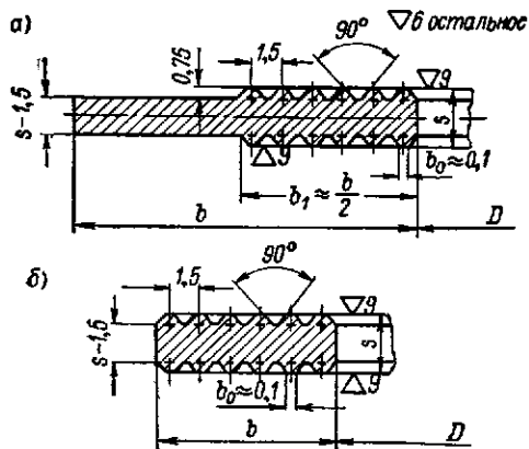
Рис. 20.2. Конструктивные элементы зубчатых (тип 3) прокладок: а — для обтюрации типа II; б — для обтюрации типа III-A. Количество зубов z зависит от величины b
