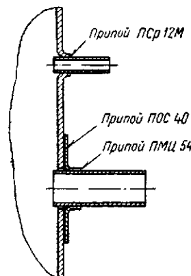
Рис. 12.10. Узел пайки патрубков и трубок к обечайкам, днищам и трубам
