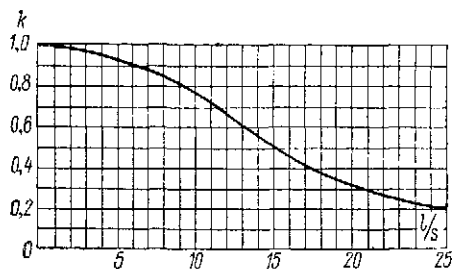
Рис. 29.2. График для определения коэффициента k в формуле (29.1)
