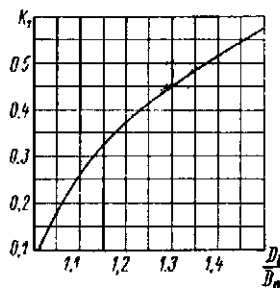
Рис. 23.5. Значения коэффициента K_1 в формуле (23.1)
