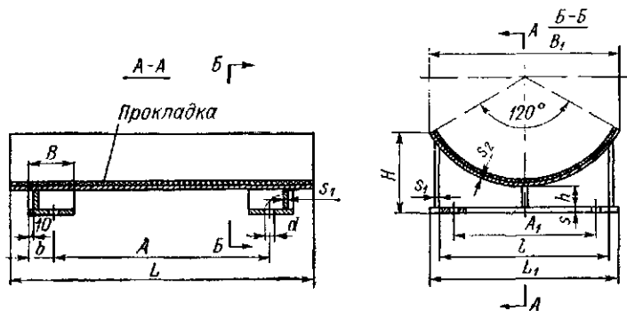
Опоры для горизонтальных цилиндрических аппаратов из винипласта (тип I по ОН 26-01-29-66)
