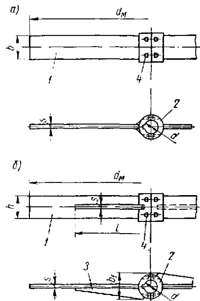
Рис. 31.4. Конструкции стальных сварных лопастных перемешивающих устройств (тип 1), шифр 10 по МН 5874—66: а — нормальное исполнение; б — усиленное исполнение; 1 — лопасть; 2 — ступица из двух половин; 3 — ребро; 4 — болты с гайками и шайбами
