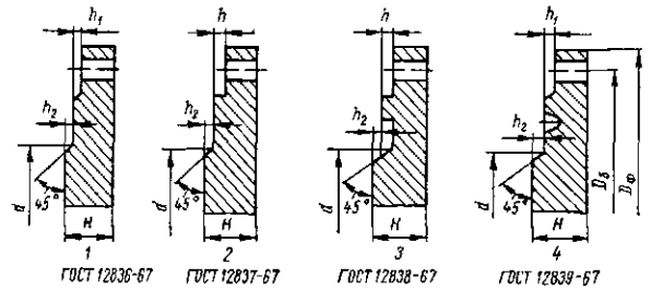
Условное обозначение заглушки с D_g = 50 \text{ мм} и p_y = 4 \text{ Мн/м}^2 (40 кгс/см 2 ) по ГОСТу 12836-67: «Заглушка 50-40 ГОСТ 12836-67»
