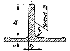
Рис. 15.21. Поперечное сечение укрепляющего ребра для плоской прямоугольной литой стенки; h_p = 5s_p ; R > 0,5s_p .
