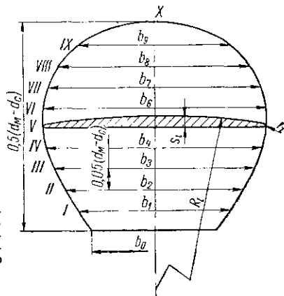
Рис. 31.10. Развертка лопасти трехлопастного пропеллерного перемешивающего устройства по МН 5874—66
