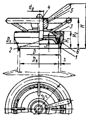
Рис. 23.20. Конструкция круглых люков с байонетным затвором и поджимным винтом для стальных аппаратов на p_y = 1,6 \text{ Мн/м}^2 (тип I по ОН 26-01-35-67)
