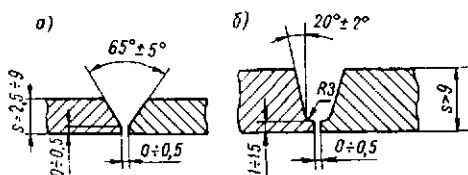
Рис. 10.6. Конструктивные элементы подготовки кромок стыковых соединений труб из стали X18H10T, 0X18H12B и X17H13M2T, свариваемых веткой ручной аргонодуговой сваркой (по ОН 26-01-71—68): а — V-образная разделка кромок; б — V-образная разделка кромок с криволинейным скосом
