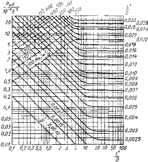
Рис. 15.4. Номограмма для расчета цилиндрических обечаек на устойчивость в пределах упругости при действии наружного давления
