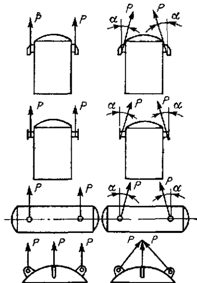
Рис. 30.1. Схемы подъема аппаратов с помощью строповых устройств по ГОСТу 13716—68
