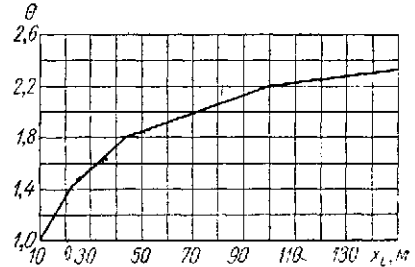
Рис. 29.15. График для определения поправочного коэффициента \theta на увеличение скоростного напора ветра для высот более 10 м
