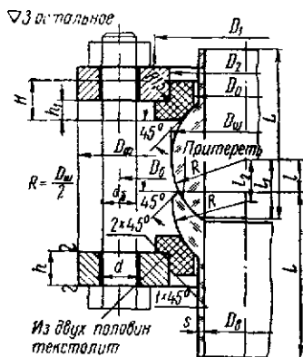
Рис. 21.18. Конструкция соединения кварцевых труб с помощью свободных фланцев
