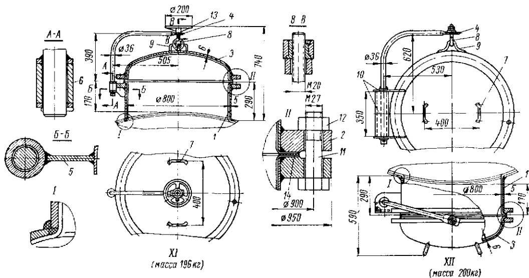
Рис. 23.14. Конструкция люков с эллиптической фланцевой крышкой и подъемно-поворотным устройством для аппаратов из углеродистой стали с внутренней химической защитой на p_y \leq 0,6 \text{ Мн/м}^2 : тип XI — для вертикальной установки, тип XII — для горизонтальной установки (по ОН 26-01-10-65)
