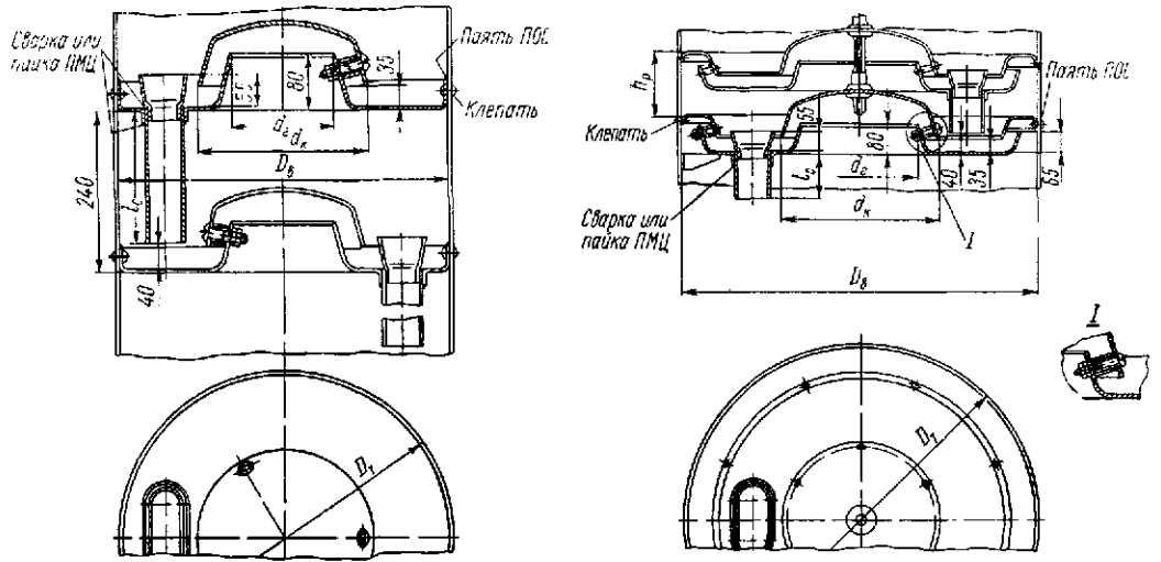
Рис. 24.8. Конструкция медных однолпачковых цельных ректификационных тарелок типа ТМО по МН 263-64 (слева) и МН 5264-64 (справа)
