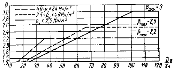
Рис. 21.11. Графики для определения коэффициента \beta в формуле (21.42). Для p_y = 10 \text{ Мн/м}^2 и \nu = 1,5
