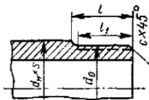
Концевые части труб в разъемных соединениях для p_y = 250 \text{ Мн/м}^2 (по данным Иркутского филиала НИИхиммаша)
