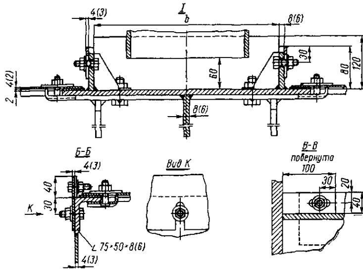
Рис. 24.14. Конструкция стальных разборных двухпоточных клапанных ректификационных тарелок по ОН 26-02-29-66
