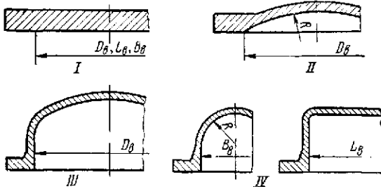
Рис. 23.1. Основные типовые конструктивные формы крышек, применяемых в химических аппаратах: I — плоская (круглая, прямоугольная, фасонная); II — сферическая (круглая); III — эллиптическая (круглая); IV — цилиндрическая (прямоугольная)
