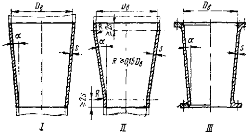
Рис. 15.28. Основные типовые конструкции конических обечайки
