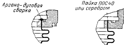
Рис. 26.2 Основные типовые конструкции присоединения сильфонов из стали марки Х18Н10Т к деталям аппарата
