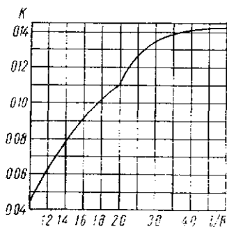
Рис. 24.18. График для определения коэффициента K в формуле (24.4) — для секции тарелки, свободно опертой по периметру
