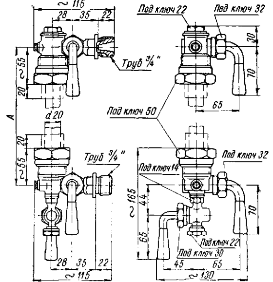
Рис. 28.1. Крановые, цапковые запорные устройства указателей уровня на p_y \leq 1,6 \text{ Мн/м}^2 по ГОСТу 9652—61
