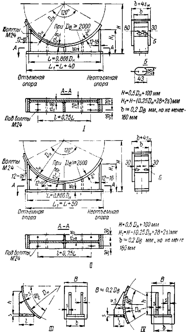
Рис. 29.9. Основные типовые конструкции опор для горизонтальных аппаратов
