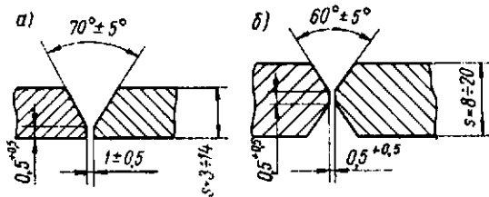
Рис. 10.11. Конструктивные элементы подготовки кромок листового титана и титановых сплавов толщиной 4—20 мм под стыковую автоматическую аргоно-дуговую сварку плавящимся электродом (по ОН 26-01-71—68): а — V-образная разделка кромок; б — X-образная разделка кромок
