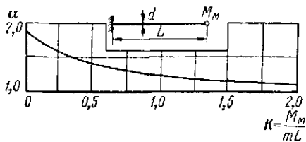
Рис. 32.3. Значение корня частотного уравнения \alpha в формуле (32.4) для расчетной схемы вала № 3
