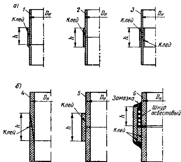
Рис. 13.2. Типовые клеевые соединения цилиндрических деталей: а — труб из металлов и сплавов; б — труб и обечаек аппаратов из неметаллических материалов; 1 и 6 — соединения внахлест; 2 и 5 — соединения встык, усиленные наружным кольцом; 3 — соединение встык, усиленное наружным и внутренним кольцом; 4 — соединение встык со скосом кромок
