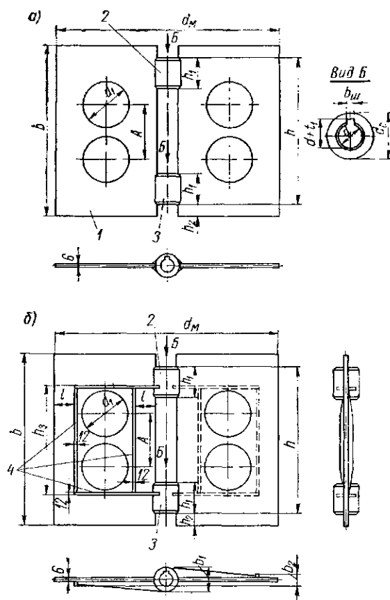
Рис. 31.5. Конструкции стальных сварных листовых перемешивающих устройств (тип 2), шифр 20 по МН 5874—66: а — нормальное исполнение; б — усиленное исполнение; 1 — лопасть; 2 — нижняя ступица; 3 — верхняя ступица; 4 — ребра
