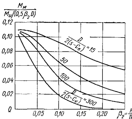
Рис. 29.3. Графики для определения отнесенного к единице длины меридионального момента M_M , действующего на стенку цилиндрического корпуса аппарата в месте присоединения к нему лапы квадратной формы
