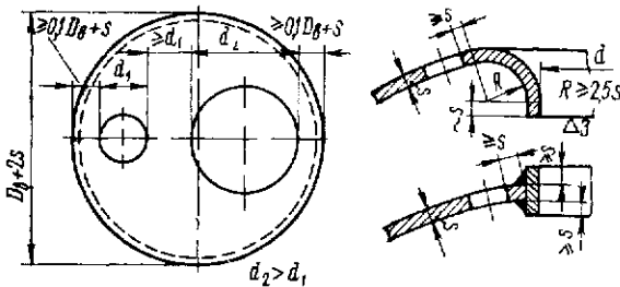
Рис. 16.3. Расположение и конструкция отверстий в эллиптических днищах
