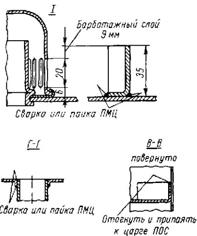
Рис. 24.6. Конструкция медных одноволочных цельных колпачковых ректификационных тарелок типа ТМК-II по МН 5259—64
