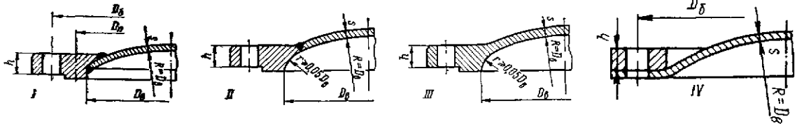
Рис. 23.9. Основные типовые конструкции сферических фланцевых крышек: I — сварные при p_y \leq 2,5 \text{ Мн/м}^2 ; II — сварные при p_y > 2,5 \text{ Мн/м}^2 ; III — кованные и литые; IV — тарельчатые (из меди) с наварными фланцами при p_y \leq 0,3 \text{ Мн/м}^2
