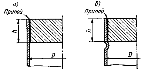
Рис. 12.7. Кольцевое соединение внахлестку тонкостенной детали с массивной: а — без препятствия для вытекания припоя; б — с гофром в тонкостенной детали, препятствующим вытеканию припоя
