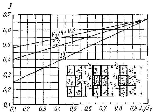
Рис. 29.20. Графики для определения коэффициента j для третьей группы ступенчатых аппаратов
