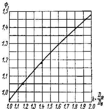
Рис. 21.8. График для определения коэффициента \Phi_1 в формуле (21.36)
