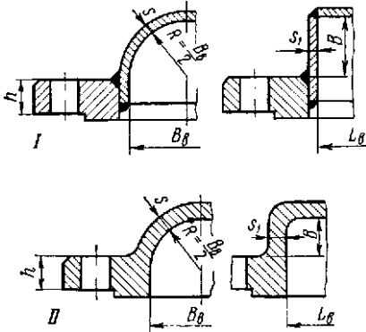
Рис. 23.15. Основные типовые конструкции фланцевых цилиндрических крышек: I — сварные; II — литые
