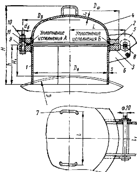
Рис. 23.12. Конструкция люков с эллиптической фланцевой крышкой и шарнирным устройством для стальных аппаратов на p_y \leq 2,5 \text{ Мн/м}^2 (типы II, III, VI и VII по ОН 26-01-10-65).
