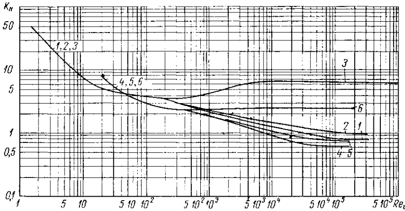
Рис. 31.3. Графики для определения критерия мощности K_N для турбинных (типы 5 и 6) перемешивающих устройств:
