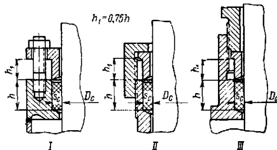
Рис. 26.4. Основные типовые конструкции сальниковых компенсаторов с мягкой набивкой, применяемых в химической аппаратуре: I — при D_c \geq 25 \text{ мм} ; II и III — при D_c < 25 \text{ мм}
