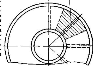
Рис. 16.16. Основные типовые конструкции кольцевых днищ в сварных аппаратах. Слева днища неукрепленные, справа — укрепленные радиальными ребрами
