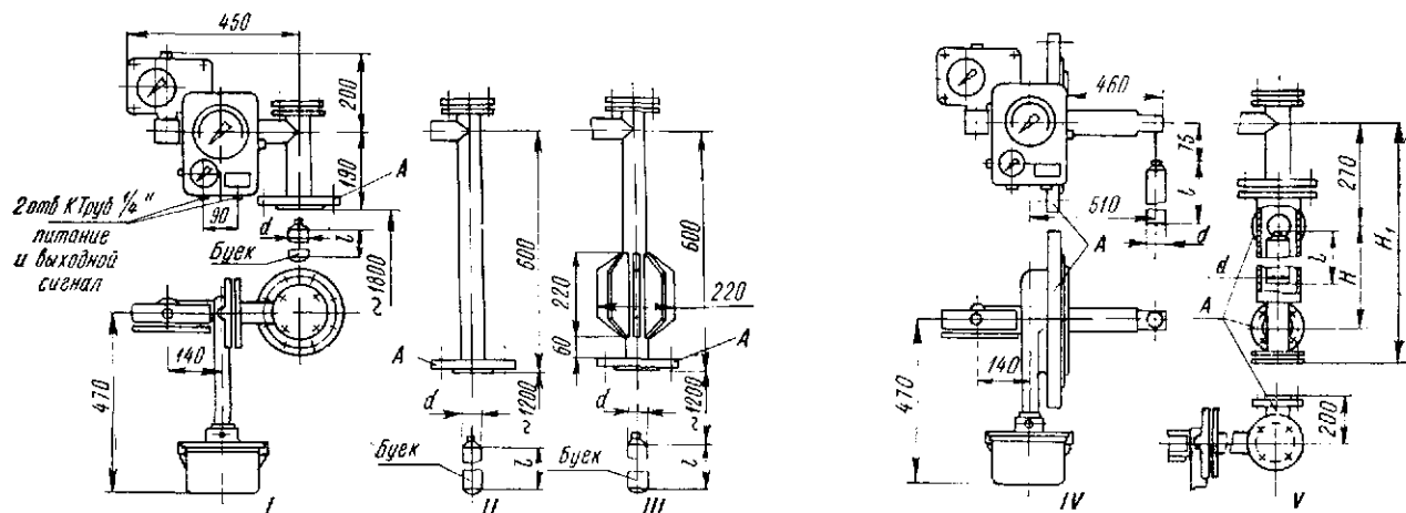
Рис. 28.7. Габариты буйкового указателя уровня (уровнемера) типа УБ на p_y = 4,0 и 6,4 \text{ Мн/м}^2 по данным рязанского завода «Теплоприбор»:
