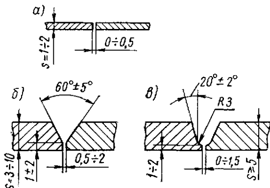
Рис. 10.2. Конструктивные элементы подготовки кромок листовой стали марки 0X17H16M3T, свариваемой ручной аргоно-дуговой сваркой неплавящимся (вольфрамовым) электродом: а — без разделки кромок; б — V-образная разделка кромок; в — V-образная разделка с криволинейным скосом кромок
