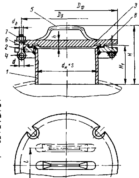
Рис. 23.3. Конструкция люков с плоской круглой фланцевой крышкой и откидными болтами для сварных аппаратов на p_y = 1,6 Мн/м 2 (тип 3 по ОН 26-01-35—67).
