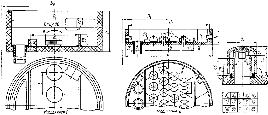
Рис. 24.10. Конструкция керамических однопоточных колпачковых ректификационных тарелок типа ТКС по ОН 26-01-11-65
