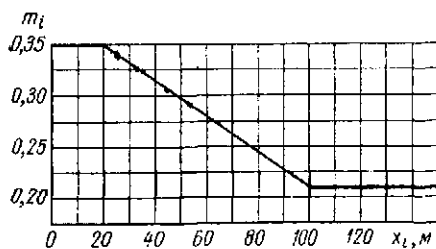
Рис. 29.17. График для определения коэффициента пульсации скоростного напора ветра m_i
