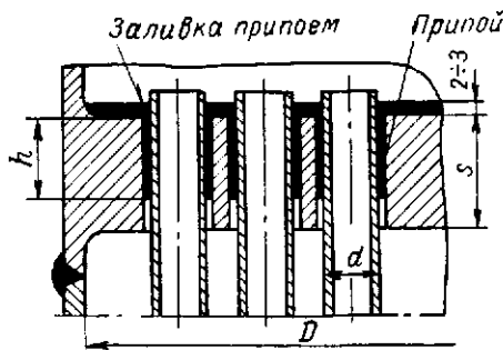
Рис. 12.9. Соединение трубок с трубной решеткой теплообменных аппаратов на мягком припое
