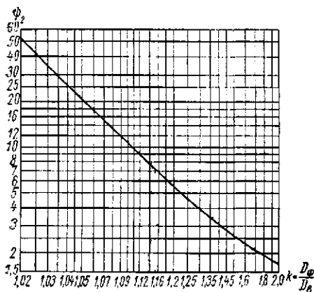
Рис. 21.9. График для определения коэффициента \Phi_2 в формуле (21.37)
