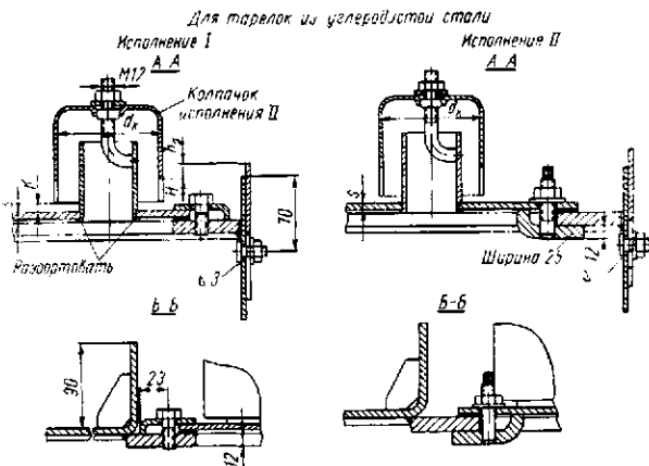
Рис. 24.2. Конструкция стальных однофазных разборных колпачковых ректификационных тарелок типа ТСК-Р по МН 5394-64
