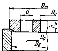
Рис. 21.20. Основные размеры свободного круглого внутреннего фланца
