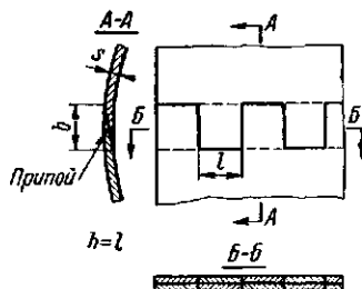
Рис. 12.3. Кольцевое соединение листового материала на твердом припое, выполненное зубец
