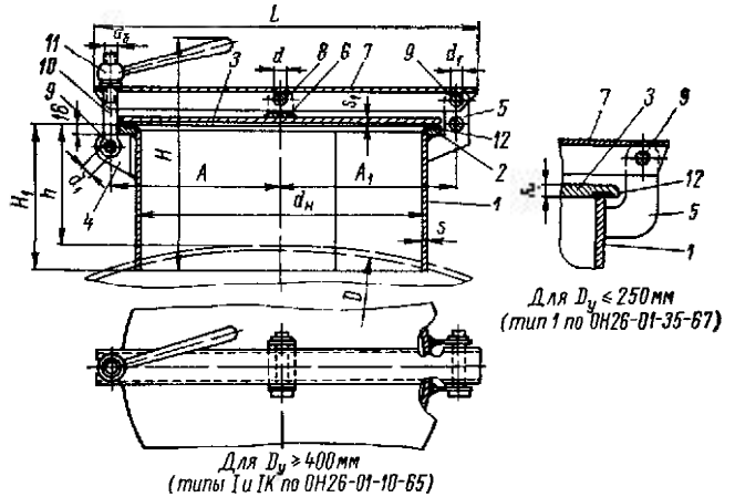
Рис. 23.17. Конструкция люков с плоской круглой крышкой и бигельным прижимным устройством для стальных аппаратов, работающих под наливом и вакуумом (типы I и IK по ОН 26-01-10—65 и тип I по ОН 26-01-35—67)
