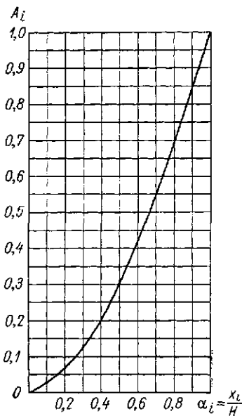
Рис. 29.21. График для определения параметра A_t .
