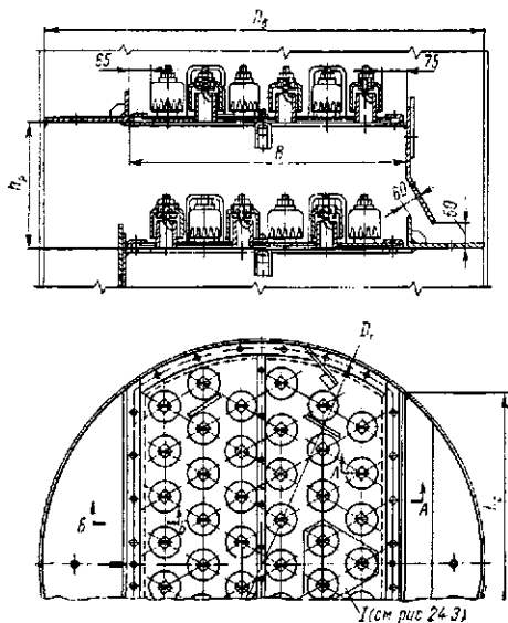
Рис. 24.2. Конструкция стальных однофазных разборных колпачковых ректификационных тарелок типа ТСК-Р по МН 5394-64
