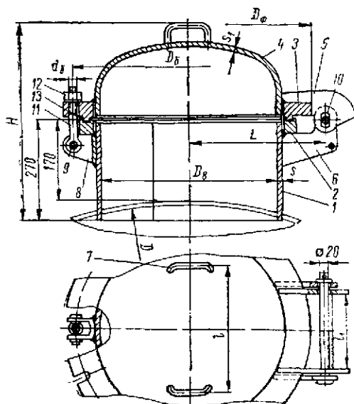
Рис. 23.11. Конструкция люков с эллиптической фланцевой крышкой, шарнирным устройством и откидными болтами для стальных аппаратов на p_y < 1,0 \text{ Мн/м}^2 (типы V и VK по ОН 26-01-10-65)
