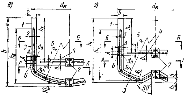
Рис. 31.6. Конструкции стальных сварных якорных перемешивающих устройств (тип 3) по МН 5874—66: а (шифр 31) и б (шифр 32) — нормальное исполнение; в (шифр 33) и г (шифр 34) — усиленное исполнение;
