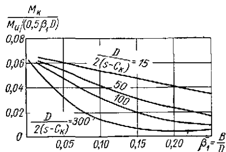
Рис. 29.4. Графики для определения отнесенного к единице длины кольцевого момента M_K , действующего на стенку цилиндрического корпуса в месте присоединения к нему лапы квадратной формы
