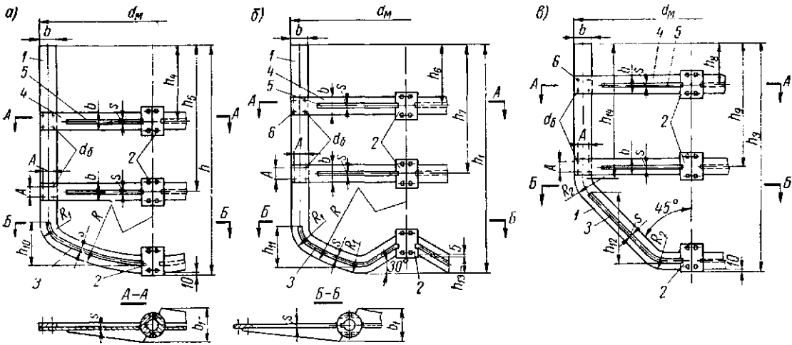
Рис. 31.7. Конструкции стальных сварных рамных перемешивающих устройств (тип 4) по МН 5874—66: а—шифр 41; б—шифр 42; в—шифр 43; 1—лопасть; 2—ступица из двух половин; 3—ребро; 4—перекладная; 5—ребро; 6—болты с гайками и шайбами
