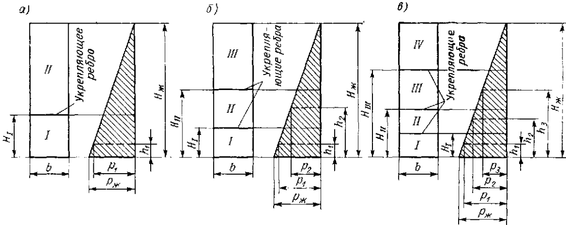
Рис 15.25. Рекомендуемое размещение укрепляющих горизонтальных ребер на вертикальных прямоугольных плоских стенках, подверженных гидростатическому давлению;
