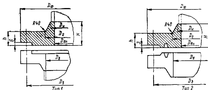
Фланцы стальных сварных аппаратов стальные цельные переходные (по данным Гипронефтемаша)
