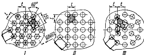
Рис. 25.3 Размещение труб в трубных решетках: I — по вершинам равносторонних треугольников; II — по вершинам квадратов; III — по концентрическим окружностям
