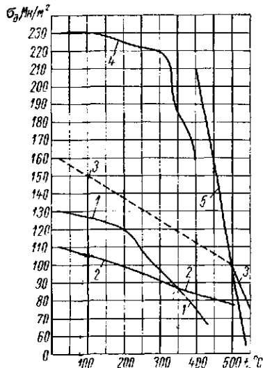
Рис. 21.3. Допускаемые напряжения на растяжение в стальных болтах диаметром d_b \geq 20 мм:
