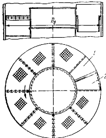
Рис. 24.16. Конструкция S-образного элемента в ректификационной тарелке с S-образными элементами
