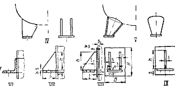
Рис. 29.1. Основные типовые конструкции опор для вертикальных аппаратов (в опорах I—III размеры 30, 40, 90 и 100 являются минимальными и действительными только для болтов М24 и М27)
