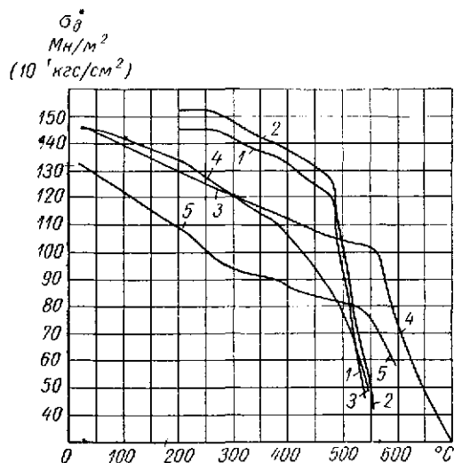
Рис. 14.2. Номинальные допускаемые напряжения \sigma_d^* для наиболее распространенных в химическом аппаратостроении марок теплоустойчивой и кислотостойкой стали. Марки стали: 1—12ХМ и 12МХ; 2—15ХМ; 3—Х5М; 4—Х18Н10Т, Х18Н12Т, Х7Н13М3Т и Х7Н13М2Т; 5—0Х18Н10Т и 0Х18Н12Т
