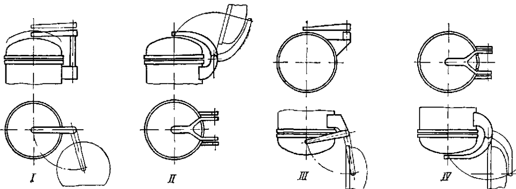
Рис. 23.23. Основные принципиальные схемы механизмов для открытия и закрытия байонетных крышек: I и II — для вертикальных крышек; III и IV — для горизонтальных крышек
