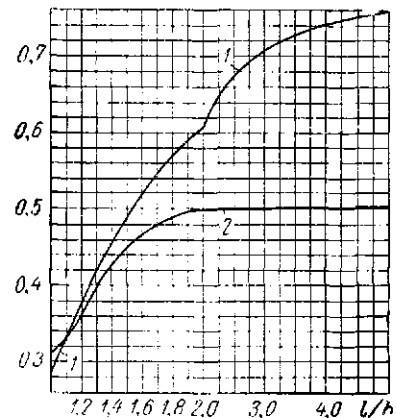
Рис. 15.22. Графики для определения коэффициента K в формуле (15.71):
