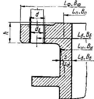
Рис. 21.15. Основные размеры цельного прямоугольного наружного фланца
