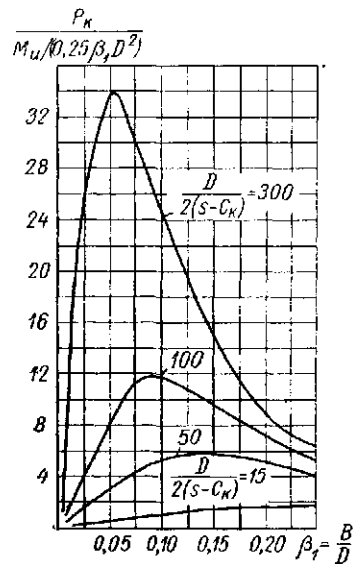
Рис. 29.6. Графики для определения относенной к единице длины кольцевой силы P_K , действующей на стенку цилиндрического корпуса в месте присоединения к нему лапы квадратной формы
