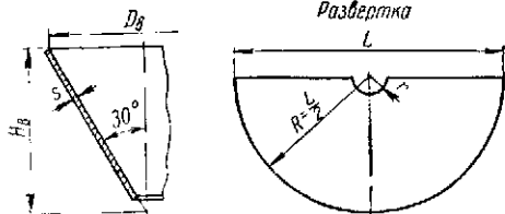
Днища конические неотбортованные с углом при вершине 60° стальные с внутренними базовыми размерами (по ГОСТу 12620—67)
