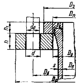
Рис. 21.19. Основные размеры свободного круглого наружного фланца с буртом
