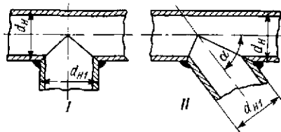
Рис. 19.4. Типовые конструкции сварного подсоединения (врезка) одной трубы к другой под углом:
