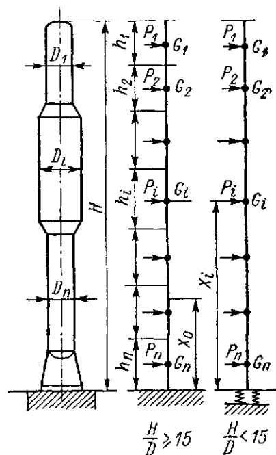
Рис. 29.13. Схема разбивки аппарата на участки при расчете его на ветровую нагрузку
