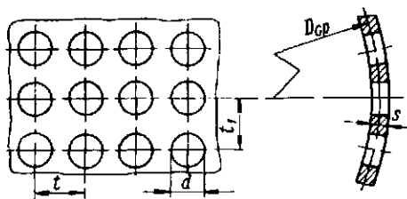
Рис. 15.1. Коридорное расположение отверстий в цилиндрической обечайке
