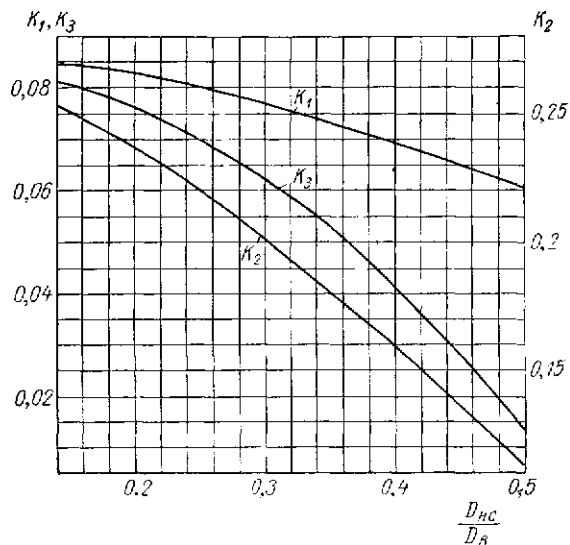
Рис. 25.6 Графики для определения коэффициентов K_1 , K_2 и K_3 в формулах (25.20) и (25.21)
