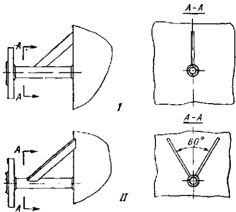
Рис. 27.1. Конструкция присоединения малых штуцеров к стенкам сварных и паяных аппаратов
