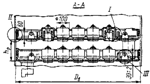
Рис. 24.4. Конструкция чугунных однопоточных цельных кольчатых ректификационных тарелок типа ГЧК по ОН 26-01-2-64
