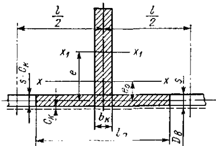
Рис. 15.6. Поперечное сечение кольца жесткости в части цилиндрической обечайки
