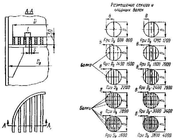
Рис. 24.19. Конструкция стальных решеток под насадку из колец Рашига диаметрами 25, 50 и 80 мм по МН 4095—62—МН 4103—62
