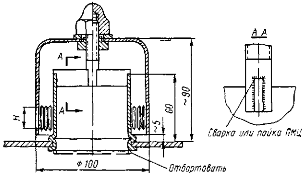
Рис. 24.5. Конструкция медных однопоточных цельных кольчатых ректификационных тарелок типа ТМК-1 по МН 5257-64
