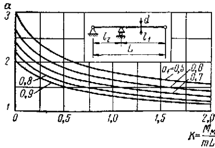
Рис. 32.2. Значение корня частотного уравнения \alpha в формуле (32.4) для расчетной схемы вала № 2
