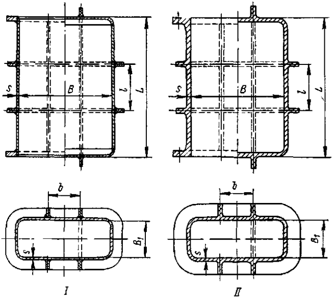
Рис. 15.19. Основные типовые конструкции коробчатых обечаек химических аппаратов: I — сварные; II — литые
