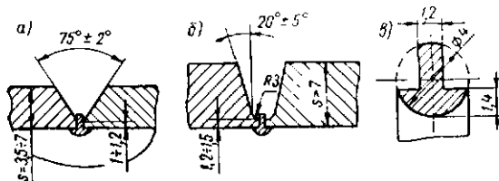
Рис. 10.5. Конструктивные элементы подготовки кромок стыковых соединений труб из стали X18H10T, 0X18H12B и X17H13M2T, выполняемых ручной аргоно-дуговой сваркой с расходными вставками (по ОН 26-01-71—68): а — V-образная разделка кромок; б — V-образная разделка кромок с криволинейным скосом; г — профиль расходного кольца
