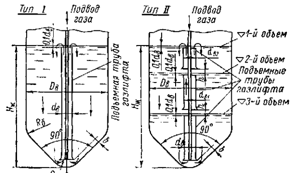
Рис. 31.12. Барботеры типа газлифта: I — для одного перемешиваемого объема; II — для нескольких перемешиваемых объемов. При D_g \leq 1,4 \text{ м} d_g = (0,08 \div 0,1) D_g ;
