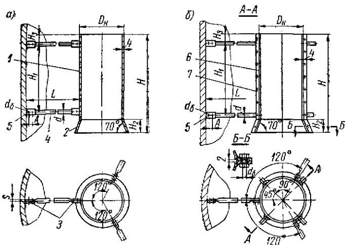
Рис. 31.11. Конструкции направляющей трубы для пропеллерных перемешивающих устройств по МН 5874—66: а — неразъемная (цельная) направляющая труба, шифр 73; б — разъемная направляющая труба, шифр 74: 1 — труба; 2 — конус; 3 — ушко; 4 — тяга; 5 — болты, гайки и шайбы; 6 — труба из четырех частей; 7 — планки для соединения четырех частей трубы между собой
