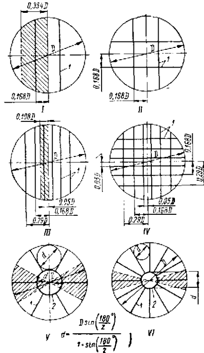
Рис. 16.15. Размещение укрепляющих ребер в плоских круглых днищах: I—IV — параллельное размещение; V и VI — радиальное размещение. Количество ребер: I — z = 2 ; II — z = 4 ; III — z = 6 ; IV — z = 12 . 1 — укрепляющее ребро; 2 — укрепляющее кольцо. При радиальном размещении ребер z \geq 6
