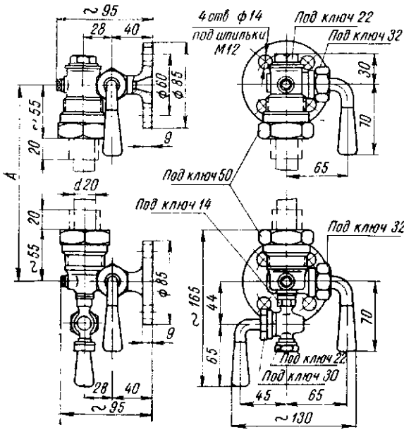
Рис. 28.2. Крановые, фланцевые запорные устройства указателей уровня на p_y = 1,6 \text{ Мн/м}^2 по ГОСТу 9652-61
