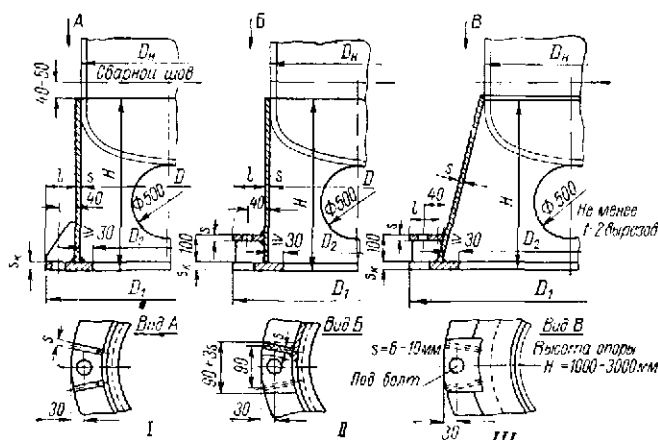
Рис. 29.1. Основные типовые конструкции опор для вертикальных аппаратов (в опорах I—III размеры 30, 40, 90 и 100 являются минимальными и действительными только для болтов М24 и М27)
