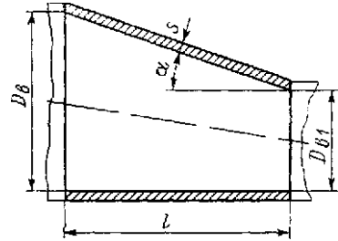
Рис. 15.29. Несимметричная коническая обечайка
