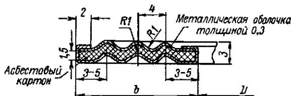
Рис. 20.3. Конструктивные элементы гофрированных (типа б) прокладок. Количество гофров z зависит от величины b
