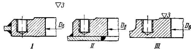
Рис. 21.22. Основные типовые конструкции фланцевых бобышек, применяемых в химическом аппаростроении: I и II—сварные; III — для литых аппаратов
