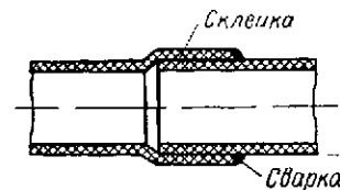
Рис. 11.1. Соединение труб из винилпласта
