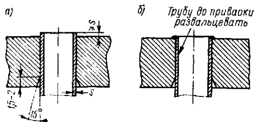
Рис. 10.13. Приварка труб к трубным решеткам стальных теплообменных аппаратов: а — подготовка кромок; б — выполненный шов
