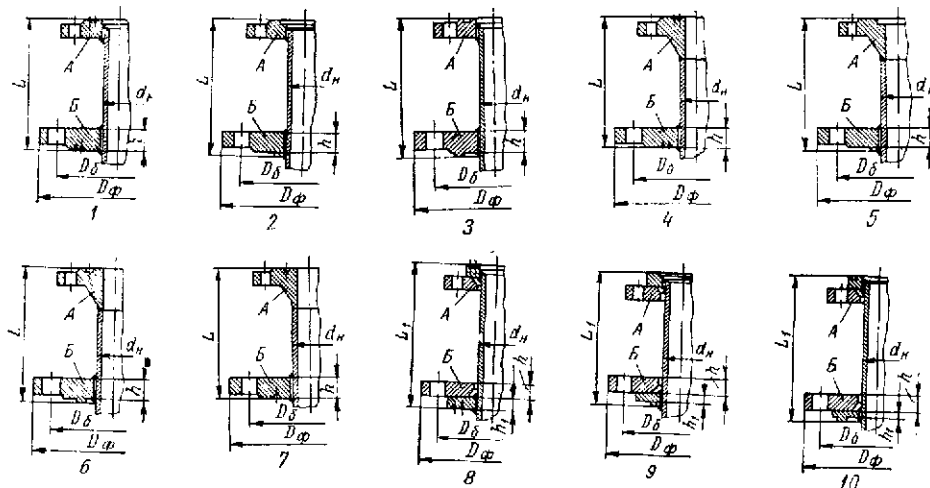
Фланцевые вводы и выводы труб в стальных сварных аппаратах на p_y \leq 6,4 \text{ Мн/м}^2 (по МН 4004—62—МН 4006—62)
