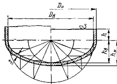
Рис. 16.1. Рекомендуемые соотношения размеров эллиптических днищ: h_б = 0,25 D_б , но не менее 0,2 D_б ; для днищ из листового проката h \geq 2s , но не менее 25 \text{ мм}
