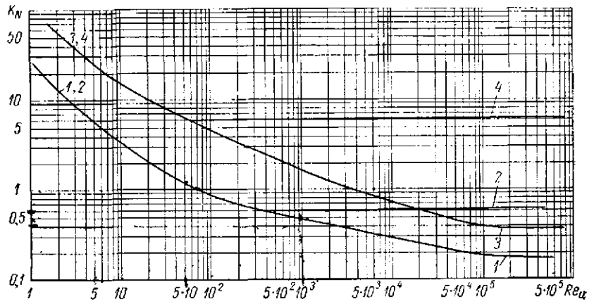
Рис. 31.1. Графики для определения критерия мощности K_N для лопастных (тип 1) и листовых (тип 2) перемешивающих устройств: 1 — для лопастных перемешивающих устройств при D_0/d_M = 1,5 ; 2 — то же, что и 1, но в аппаратах с перегородками; 3 — для листовых перемешивающих устройств при D_0/d_M = 2 ; 4 — то же, что и 3, но в аппаратах с перегородками
