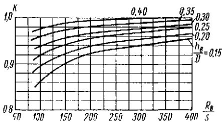
Рис. 16.5. График для определения коэффициента K в формуле (16.8)
