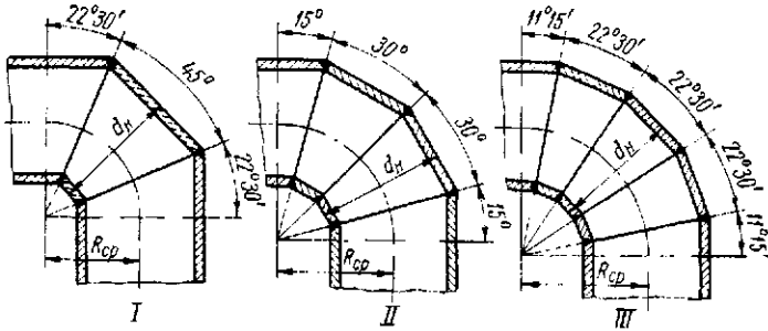
Рис. 19.1. Основные типовые конструкции сварных секторных отводов с углом поворота 90°: I — при R_{ср} \geq 0,75 d_{н} ; II — при R_{ср} \geq 0,9 d_{н} ; III — при R_{ср} \geq d_{н}
