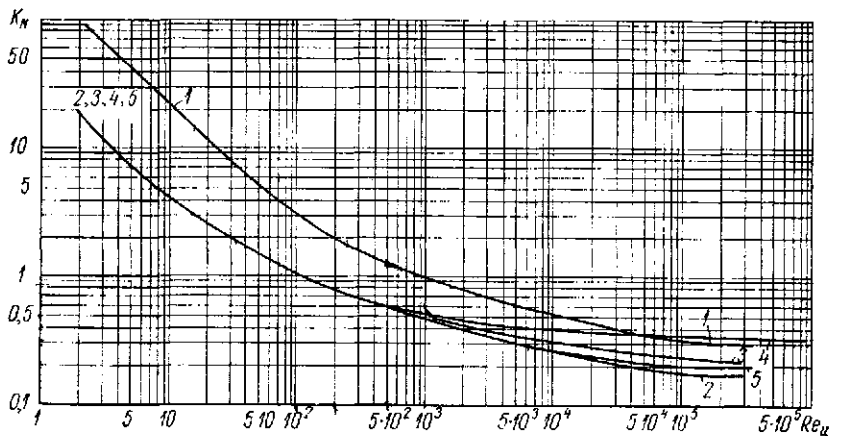
Рис. 31.2. Графики для определения критерия мощности K_N для якорных (тип 3), рамных (тип 4) и пропеллерных (тип 7) перемешивающих устройств: 1 — для якорных и рамных перемешивающих устройств при D_0/d_M = 1,5 ; 2 — для пропеллерных перемешивающих устройств при D_0/d_M = 3 ; 3 — то же, что и 2, но при D_0/d_M = 4 ; 4 — то же, что 2 и 3, но в аппаратах с перегородками; 5 — то же, что 2 и 3, с направляющей трубой
