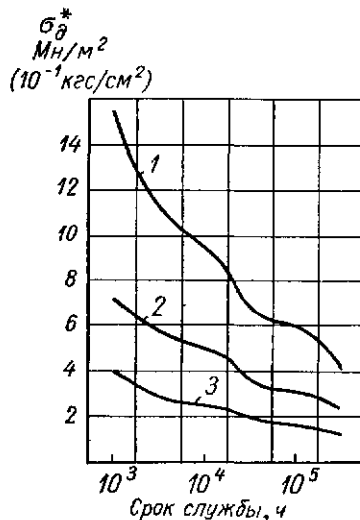
Рис. 14.3. Номинальные допускаемые напряжения \sigma_{\partial}^* для винилпласта в зависимости от срока службы и расчетной температуры. При расчетной температуре: 1 — 20° С; 2 — 40° С; 3 — 60° С
