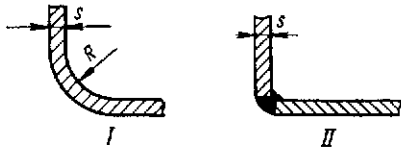
Рис. 15.18. Сопряжение под углом плоских прямоугольных стенок: I — для стенок из листов R \geq 5s ; для литых стенок R > 2s ; II — допускаемое для сварных аппаратов, работающих под наливом
