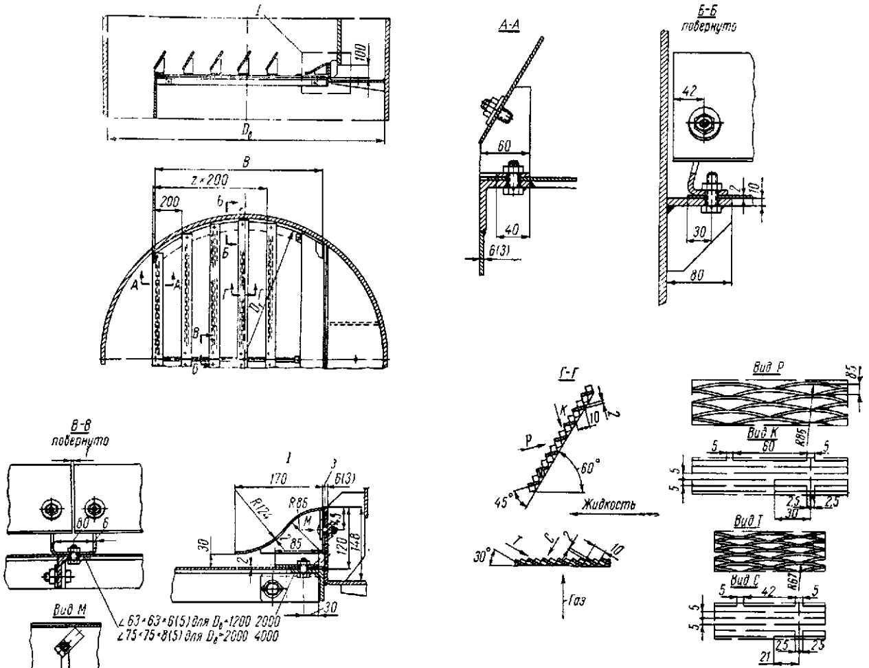
Рис. 24.11. Конструкция стальных однопоточных разборных ситчатых с отбойными элементами ректификационных тарелок по ОН 26 02-36-66
