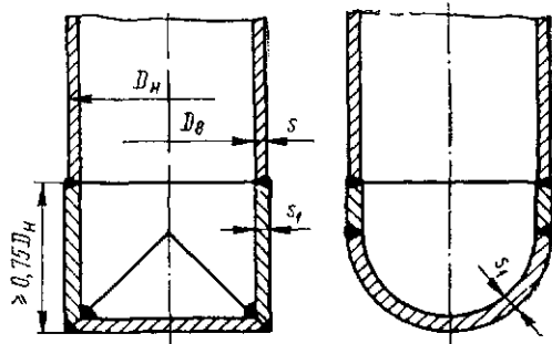
Рис. 16.17. Конструкция цилиндрического днища в сварных аппаратах. Справа при базовом D_0' , слева — при базовом D_n .
