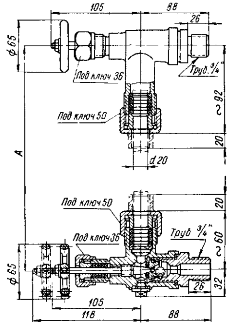
Рис. 28.4. Вентильные, цапковые запорные устройства указателей уровня на p_y = 4,0 \text{ Мн/м}^2 по ГОСТу 9652-61
