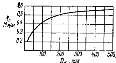
Рис. 20.4. График для определения удель- ной нагрузки по линии уплотнения q_\lambda в формуле (20.3)
