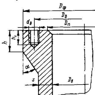
Рис. 21.13. Основные размеры цельнокованого фланца (пневматического или заводского аппарата) для p_y > 10 \text{ Мн/м}^2 . h = h_1 + 0,5 d_0 при \alpha = 30^\circ ; h = h_1 + d_0 при \alpha = 45^\circ
