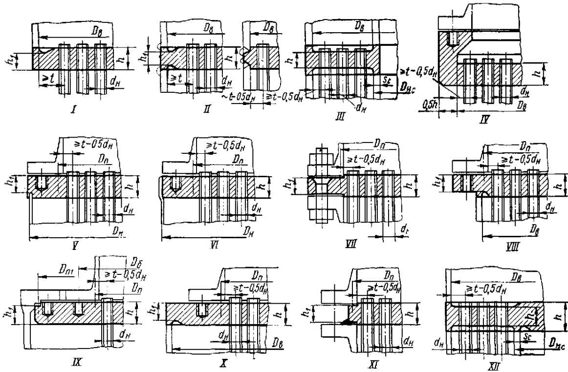
Рис. 25.1 Основные типовые конструкции плоских трубных решеток, применяемых в химическом аппаратостроении
