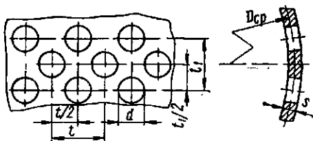
Рис. 15.2. Шахматное расположение отверстий в цилиндрической обечайке
