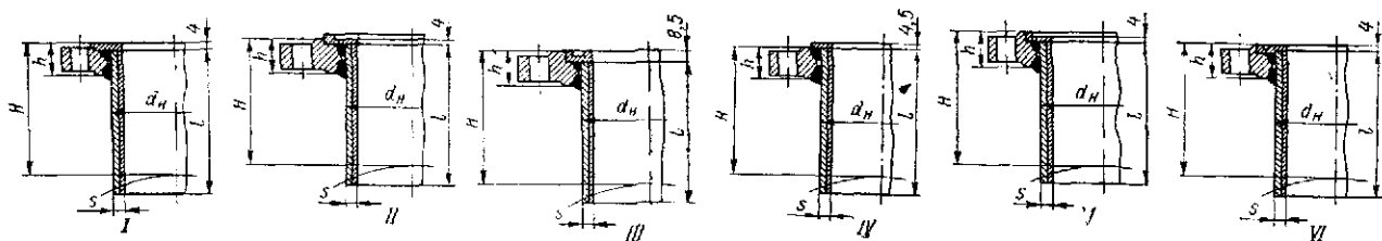
Штуцера из двухслойной стали с приварными фланцами и наплавленной уплотнительной поверхностью на p_y \leq 6,4 Мн/м 2 (по МН 4579—63—МН 4584—63)
