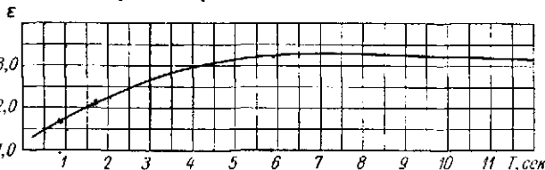
Рис. 29.16. График для определения коэффициента динамичности \epsilon
