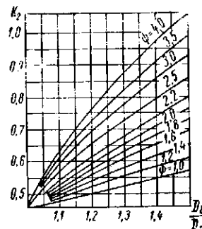
Рис. 23.6. Значения коэффициента K_2 в формуле (23.3)
