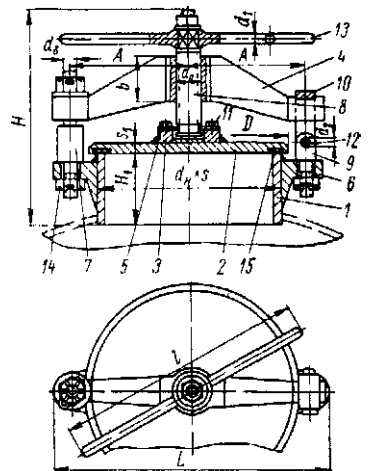
Рис. 23.18. Конструкция люков с плоской круглой крышкой и бигельным прижимным устройством для стальных аппаратов на p_y < 0,6 \text{ Мн/м}^2 (тип 2 по О 26-01-35—67)
