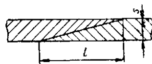
Рис. 12.2. Паяное соединение встык листового материала со скосом кромок
