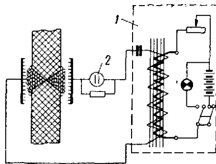
Рис. 11.5. Схема электронискрового дефектоскопа
