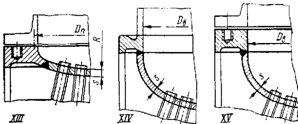
Рис. 25.2 Основные типовые конструкции сферических и эллиптических трубных решеток, применяемых в химическом аппаратостроении: XIII — сферическая; XIV и XV — эллиптические
