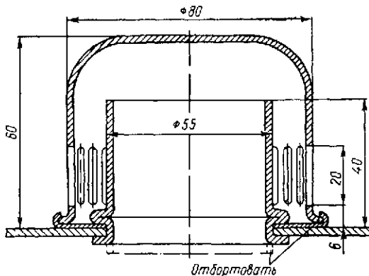
Рис. 24.7. Конструкция медных одноволочных цельных колпачковых ректификационных тарелок типа ТМК-III по МН 5261—64
