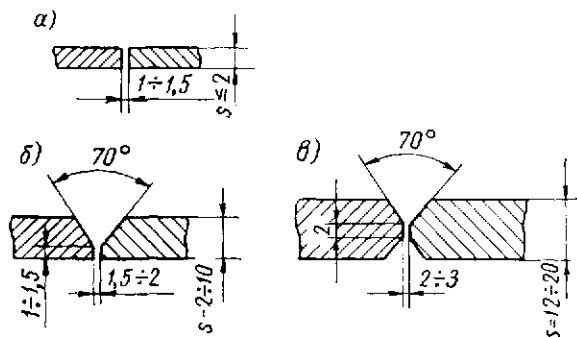
Рис. 10.8. Конструктивные элементы подготовки кромок листового латуни марки Л62, свариваемой встык газовой сваркой (по ОН 26-01-71—68): а — без скоса кромок; б — V-образная разделка кромок; в — X-образная разделка кромок
