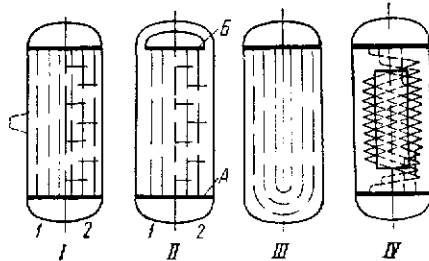
Рис. 25.4 Основные конструктивные схемы цилиндрических кожухотрубных теплообменников с плоскими трубными решетками: I — прямотрубный жесткой конструкции и жесткой (с компенсатором на корпусе); 1 — без перегородок; 2 — с перегородками; II — с плавающей головкой; III — с U-образными трубами; IV — с витыми трубами и сердечником, жестко соединенным с трубными решетками
