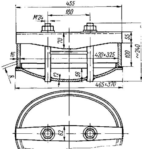
Рис. 23.16. Конструкция овального люка из углеродистой стали с внутренней съемной бигельной крышкой на p_y < 0,8 \text{ Мн/м}^2 ; масса 35,6 кг (тип VIII по МХ 43—56)
