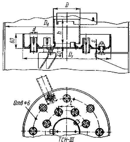
Рис. 24.21. Конструкция стальных насадочных тарелок типов ТСН-II и ТСН-III по ОН 26 01 15—65
