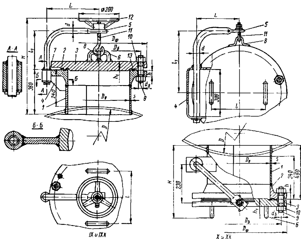
Рис. 23.4. Конструкция люков с плоской круглой фланцевой крышкой в подъемно-поворотном устройстве для сварных аппаратов на p_y = 4 Мн/м 2 (типы IX, IXK, X и XK по ОН 26-01-10—65).
