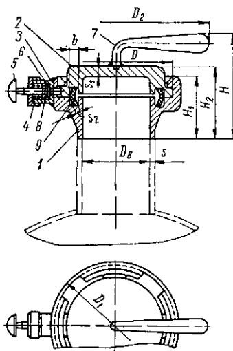
Рис. 23.21. Конструкция круглых люков с байонетным затвором для стальных аппаратов на p_y = 1,6 \text{ Мн/м}^2 (тип 3 по ОН 26-01-35-67)
