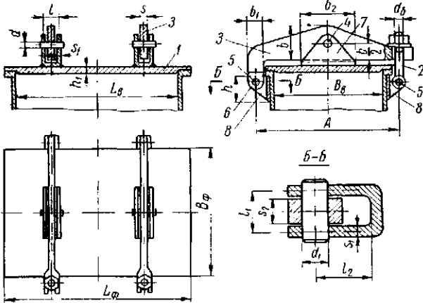
Рис. 23.19. Конструкция плоской прямоугольной крышки с двумя бигельными устройствами:
