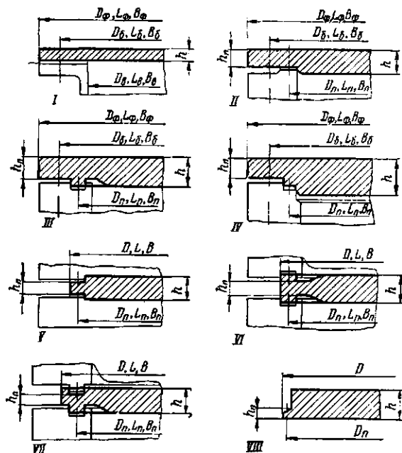
Рис. 23.2. Основные типовые конструкции плоских фланцевых крышек: I—IV — цельные круглые и прямоугольные фланцевые крышки; V—VII — закладные между фланцами круглые и прямоугольные крышки (заглушки); VIII — закладная круглая крышка для аппаратов высокого давления
