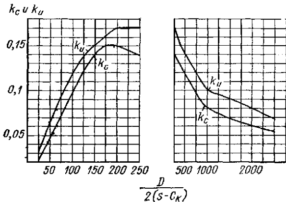
Рис. 15.8. График для определения коэффициентов k_c и k_u в формулах (15.38) и (15.47)
