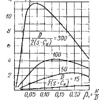
Рис. 29.5 Графики для определения относенной к единице длины меридиональной силы P_m , действующей на стенку цилиндрического корпуса в месте присоединения к нему лапы квадратной формы
