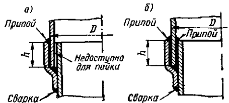
Рис. 12.5. Кольцевое соединение деталей примерно одинаковой толщины, выполненное вназ: а — при односторонней пропайке; б — при двухсторонней пропайке
