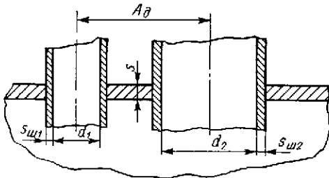
Рис. 18.4. Размещение двух смежных штуцеров
