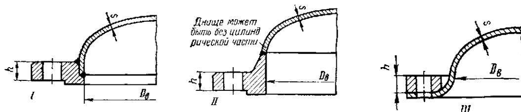
Рис. 23.10. Основные типовые конструкции эллиптических фланцевых крышек: I — сварные стальные при p_y < 2,5 \text{ Мн/м}^2 и из цветных металлов при p_y < 0,6 \text{ Мн/м}^2 ; II — сварные стальные при p_y > 2,5 \text{ Мн/м}^2 и из цветных металлов при p_y > 0,6 \text{ Мн/м}^2 ; III — из меди с наварными фланцами при p_y < 0,3 \text{ Мн/м}^2
