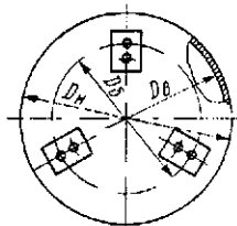
Привязочные размеры опор (стоек) в вертикальных цилиндрических аппаратах (по ОН 26-01-69—68)
