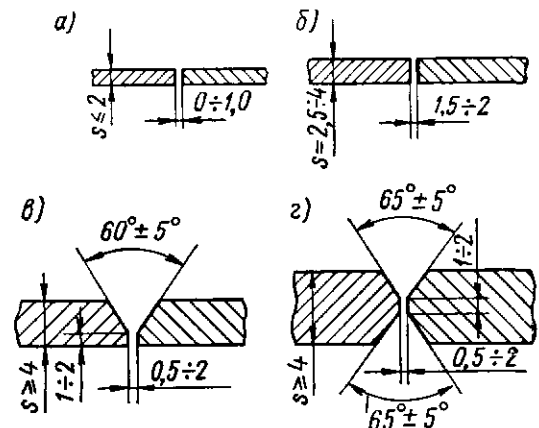
Рис. 10.1. Конструктивные элементы подготовки кромок листовой стали марок 0X18H10T и X18H10T, свариваемой ручной аргоно-дуговой сваркой неплавящимся (вольфрамовым) электродом: а и б — без скоса кромок; в — V-образная разделка кромок; г — X-образная разделка кромок
