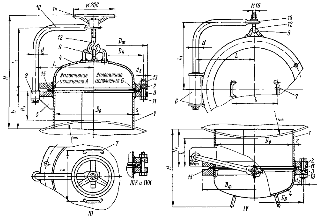
Рис. 23.13. Конструкция люков с эллиптической фланцевой крышкой и подъемно-поворотным устройством для стальных аппаратов на p_y \leq 2,5 \text{ Мн/м}^2 (типы III, IIIK; IV и IVK по ОН 26-01-10-65)
