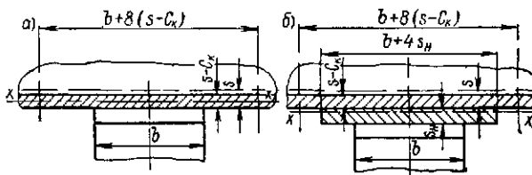
Рис. 29.11. Расчетные сечения стенки горизонтального цилиндрического корпуса в месте опоры при расчете его на прочность и устойчивость от действия реакции опоры: а — сечение неукрепленной стенки; б — сечение стенки, укрепленной накладкой
