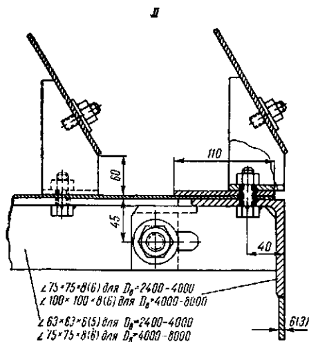
Рис. 24.12. Конструкция стальных двухпоточных разборных ситчатых с отбойными элементами ректификационных тарелок по ОН 26-02-30-66: А — исполнение III; Б — исполнение IV
