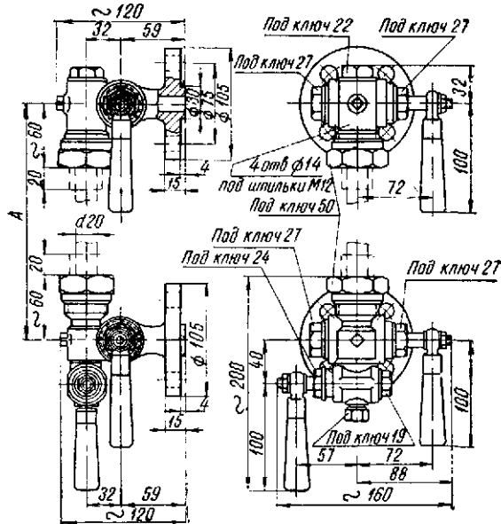
Рис. 28.3. Крановые, фланцевые запорные устройства указателей уровня на p_y = 2,5 \text{ Мн/м}^2 по ГОСТу 9652-61
