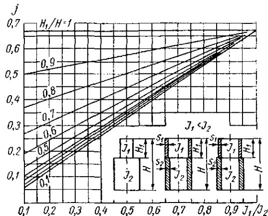
Рис. 29.18. График для определения коэффициента j для первой группы ступенчатых аппаратов
