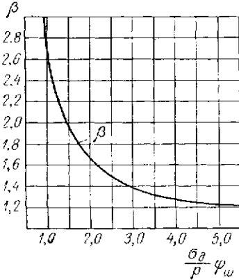
Рис. 15.14. График для определения коэффициента толстостенности обечайки β в формулах (15.57) и (15.58)
