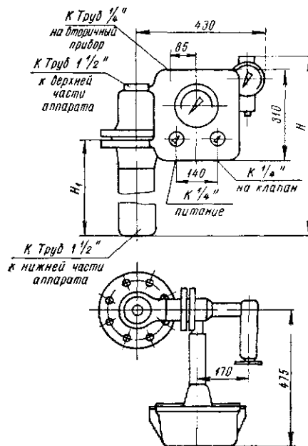
Рис. 28.8. Габариты буйкового регулятора уровня типа РУКЦ на p_y \leq 6,4 \text{ Мн/м}^2 по данным завода «Леннефтекип». Высоты H и H_1 зависят от пределов регулирования и соответственно равны: для пределов регулирования 400 мм H = 680 \text{ мм} и H_1 = 400 \text{ мм} ; для пределов регулирования 800 мм H = 1080 \text{ мм} и H_1 = 800 \text{ мм} .
