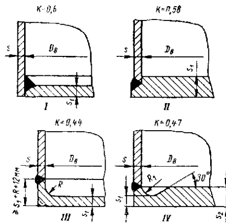
Рис. 16.12. Основные типовые конструкции плоских круглых днищ для аппаратов, работающих под избыточным давлением. R \geq 2,5 s ; R_1 \leq 0,15 s_1 , но не менее 8 и не более 20 мм; для типа IV s_1 = (0,6 - 0,8) s
