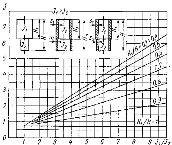
Рис. 29.19. Графики для определения коэффициента j для второй группы ступенчатых аппаратов
