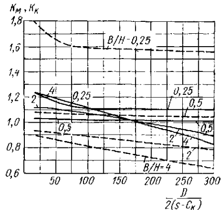
Рис. 29.7. Графики для определения коэффициента K в формуле (29.3), — — — — K_m ; — — — — K_K
