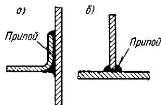
Рис. 12.12. Узел пайки гарни- туры к корпусу аппарата при соединении: а — внахлестку; б — втавр
