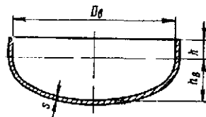
Днища эллиптические отбортованные стальные с внутренними базовыми размерами (по ГОСТу 6533—68)
