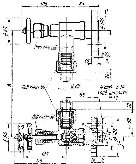
Рис. 28.5. Вентильные, фланцевые запорные устройства указателей уровня на p_y = 4,0 \text{ Мн/м}^2 по ГОСТу 9652-61
