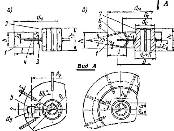
Рис. 31.8. Конструкции стальных сварных турбинных перемешивающих устройств (типы а и б) по МН 5874—66: а — тип а (шифр 50), открытые; б — тип б (шифр 60), закрытые; 1 — лопасть; 2 — ступица из двух половин; 3 — диск из двух половин; 4 — планка; 5 — болты с гайками и шайбами; 6 — диск; 7 — ступица; 8 — конус
