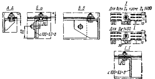
Рис. 24.15. Конструкция стальных разборных решетчатых ректификационных тарелок по Н 964-63 Гипрокефтемаш
