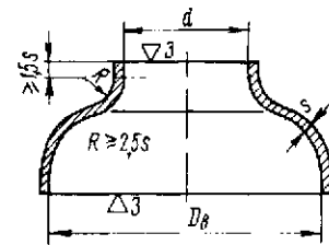
Рис. 16.4. Конструкция отверстия в эллиптических днищах при d > 0,5D_n
