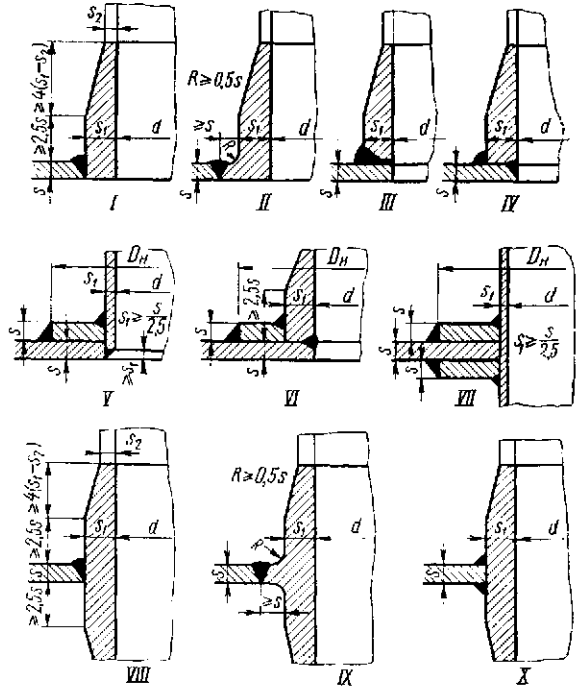
Рис. 18.1 Основные типовые конструкции укрепления отверстий для приварных штуцеров и труб в сварной аппаратуре (из пластичных материалов), работающей при статических нагрузках. Укрепление присоединяемых труб: I—IV — втулочное; V — накладочное; VI — втулочно-накладочное. Укрепление ввода труб: VII — накладочное; VIII—X — втулочное
