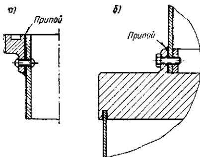
Рис. 12.8. Плотно-прочные болтовые (винтовые) или заклепочные соединения деталей на мягком припое: а — присоединение бурта к трубе на заклепках; б — присоединение обечайки к трубной доске на болтах (винтах)
