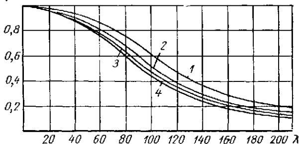
Рис. 15.9. График для определения коэффициента уменьшения допускаемых напряжений при продольном изгибе центрально сжатых элементов \varphi в формуле (15.41). Для стали марок: 1 — Ст. 3, 10, 20, 20К; 2 — 12ХМ, 12МХ, 15ХМ, Х5М; 3 — 16ГС, 09Г2С; 4 — Х18Н10Т, 0Х18Н10Т, Х18Н12Т, 0Х18Н12Т, Х17Н13М2Т, Х17Н13М3Т
